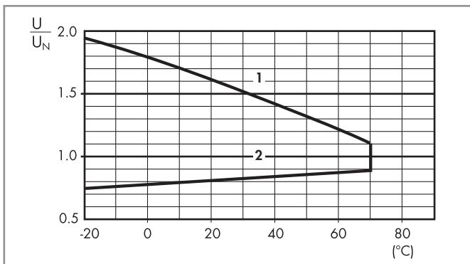
R 59 - Campo de funcionamiento de la bobina DC en función de la temperatura ambiente
